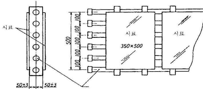
그림 6 - 형광등의 배치
