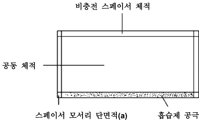
그림 X1.2 비충전 스페이서 체적
