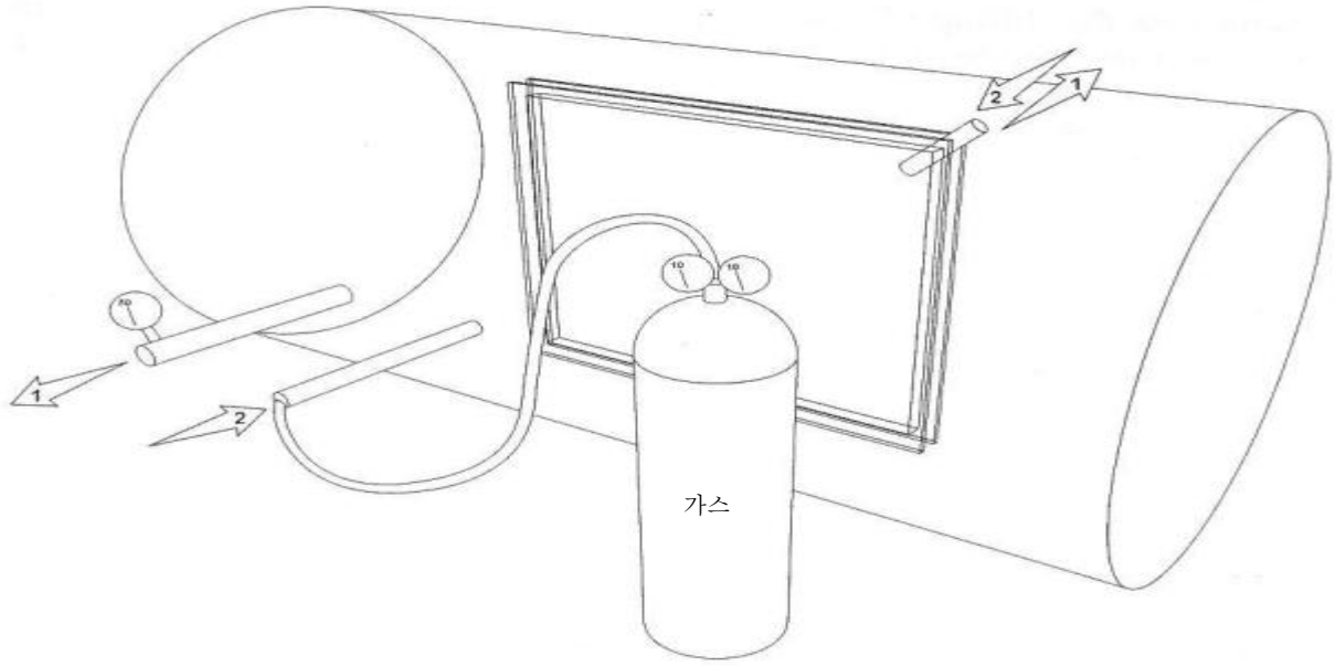
그림 2- 챔버 내에서의 가스 주입 방법
