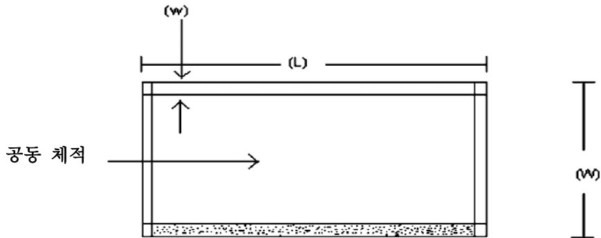
그림 X1.1 가스주입 단열유리 치수
