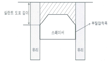
그림 4-봉착 상태
